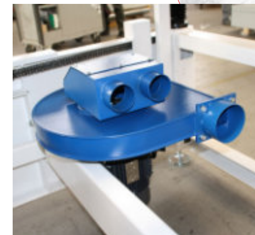
Wewnętrzny wentylator podciśnienia (zmiennie ustawienie, falownik) Internal vacuum fan (setting variable, inverter) Ventilateur dépression à l'intérieur (réglage variable, inverter)
