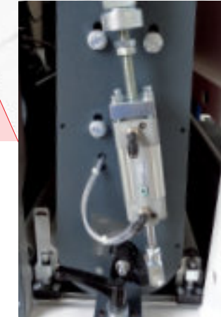
Pneumatyczny system on-off On-off pneumatic system Système on-off pneumatique
